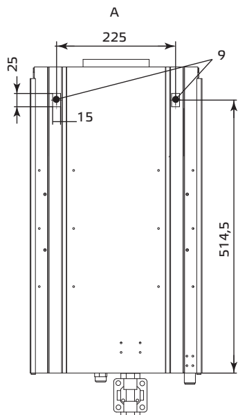
Рисунок 1 — Водонагреватель проточный газовый. Внешний вид, габаритные и монтажные размеры
